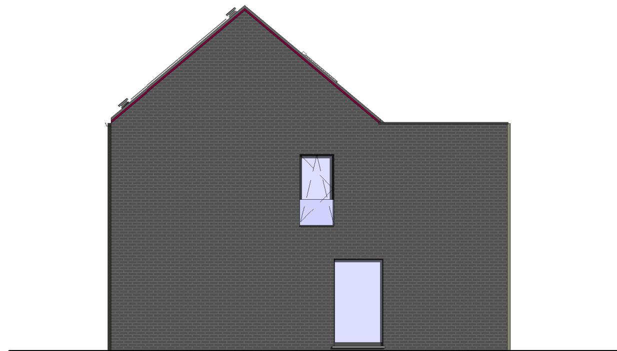
linkergevel
