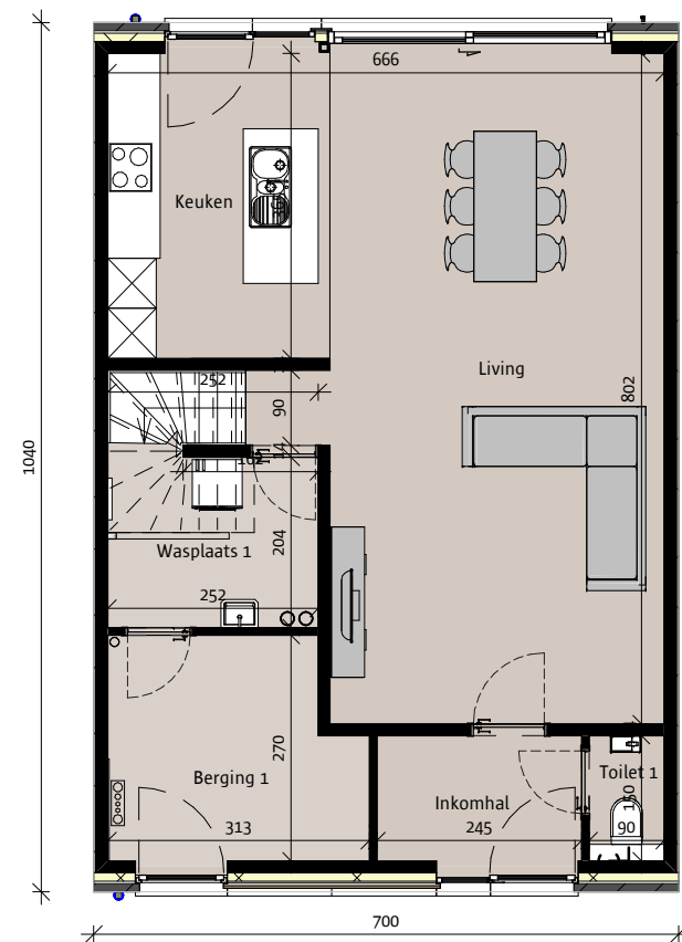
gelijkvloers Opp. 72.8 m 2
