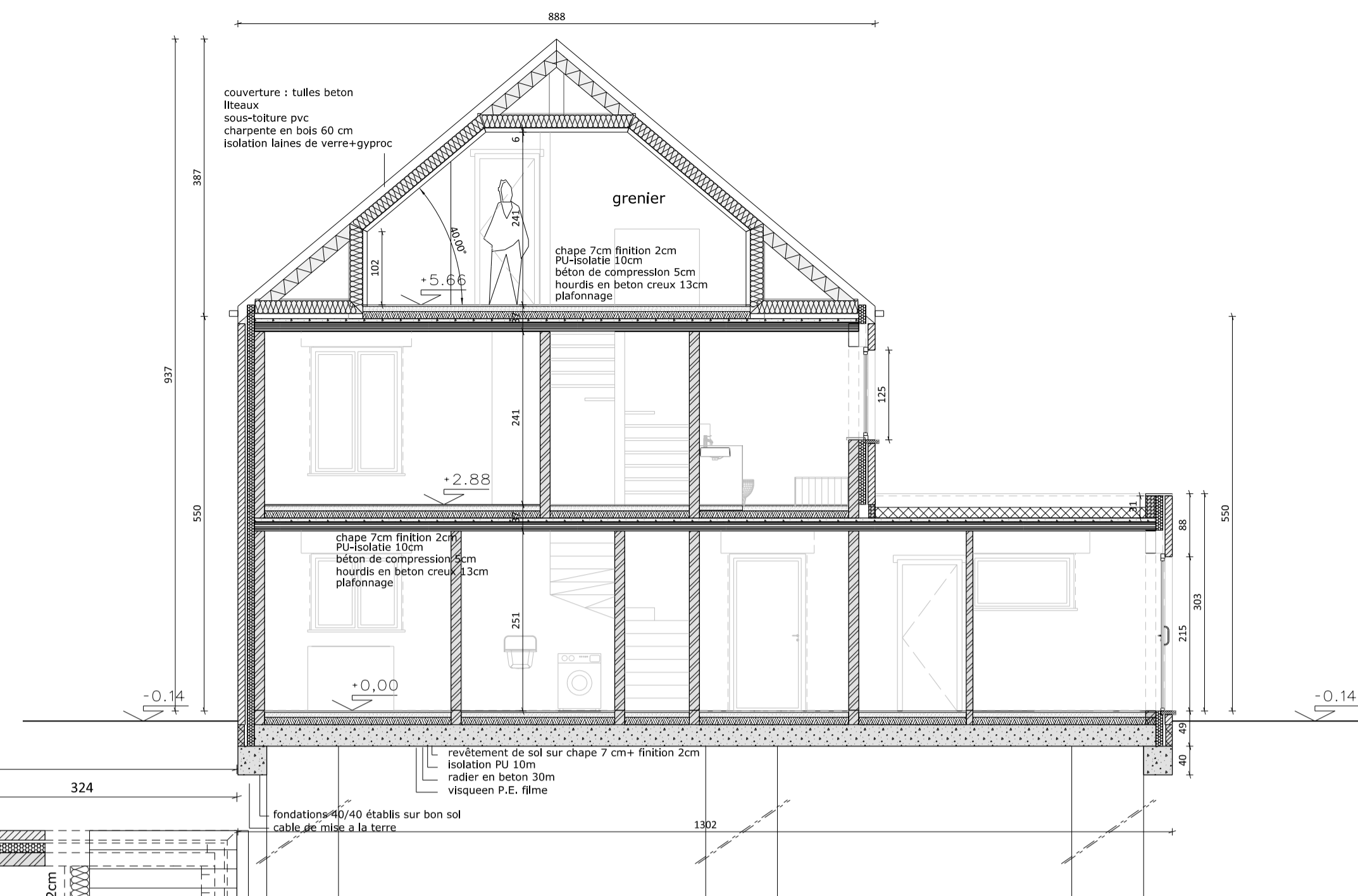
COUPE
