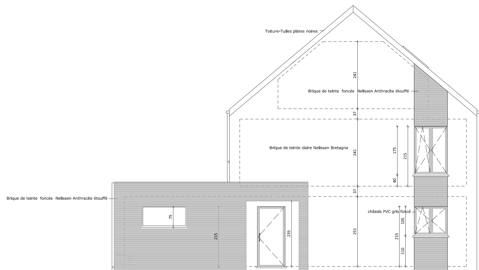
FACADE AVANT
