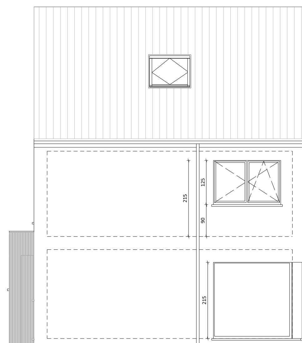
FACADE DROITE
