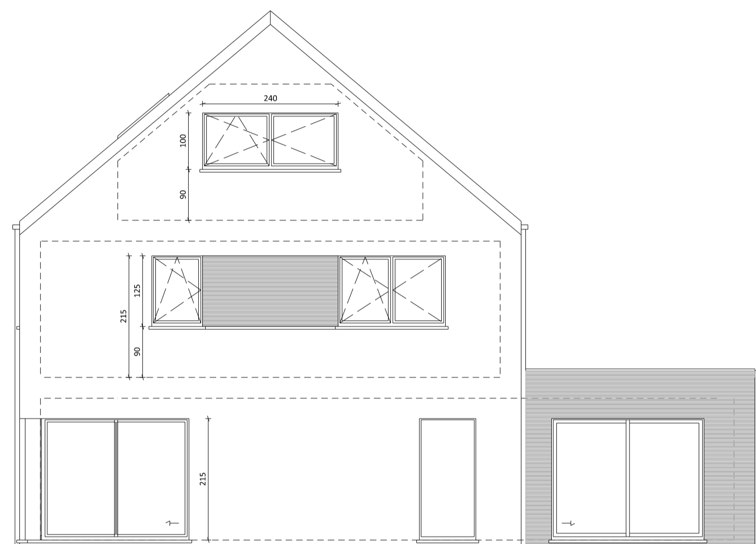
FACADE AVANT
