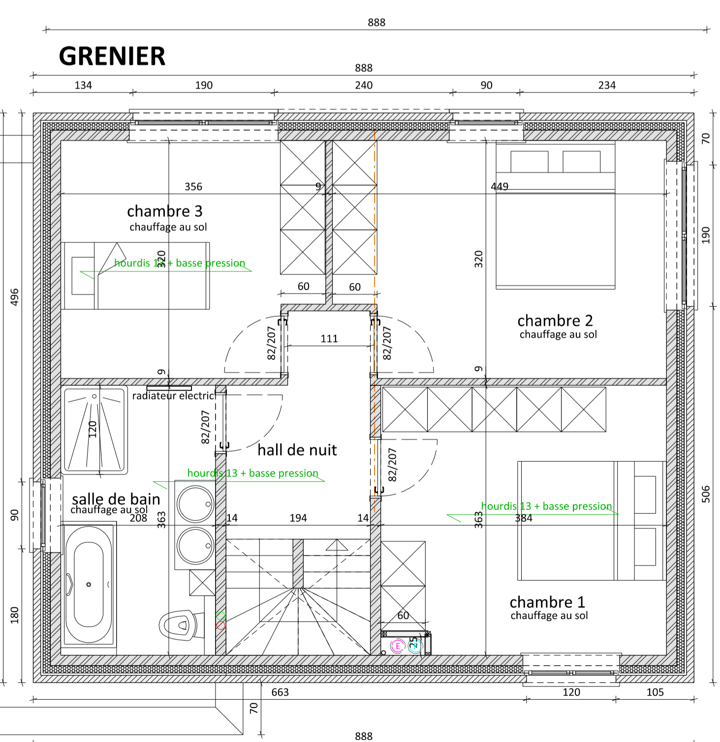
ETAGE
