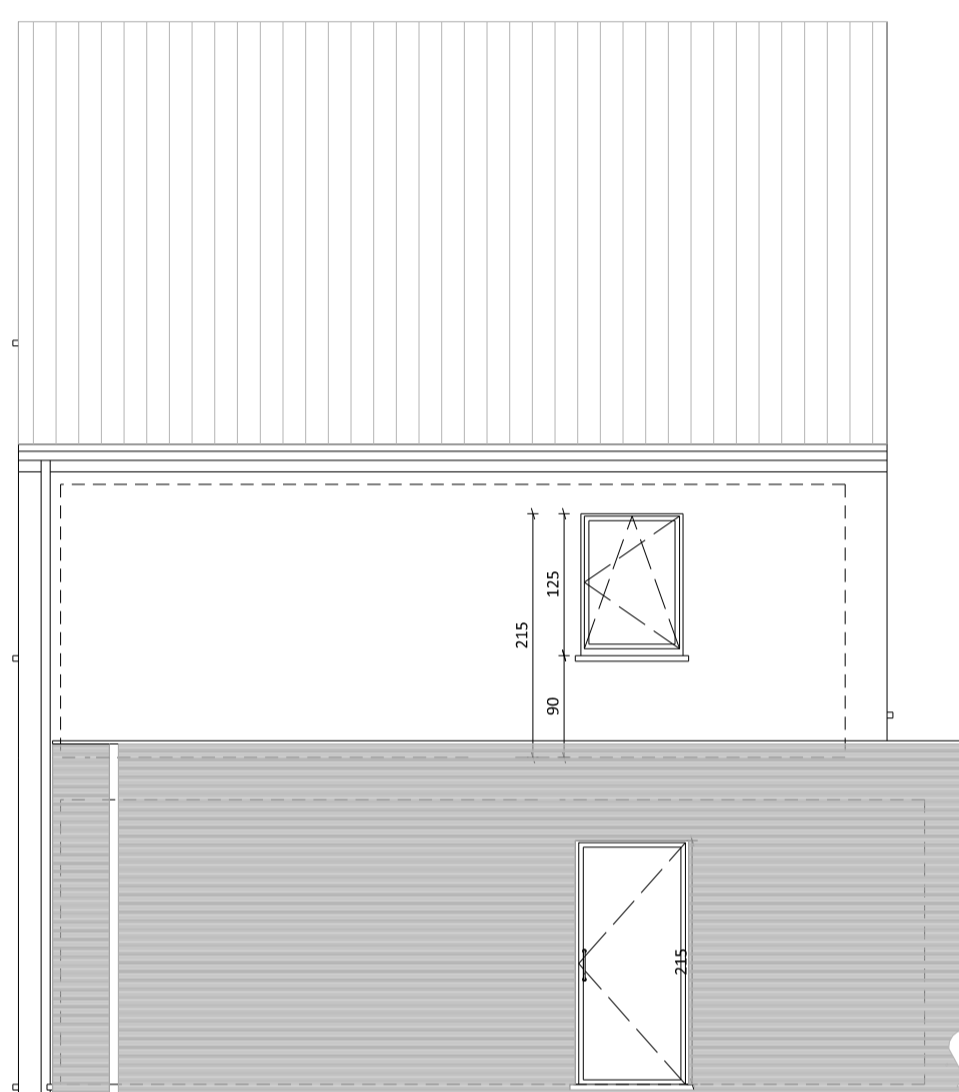
FACADE DROITE
