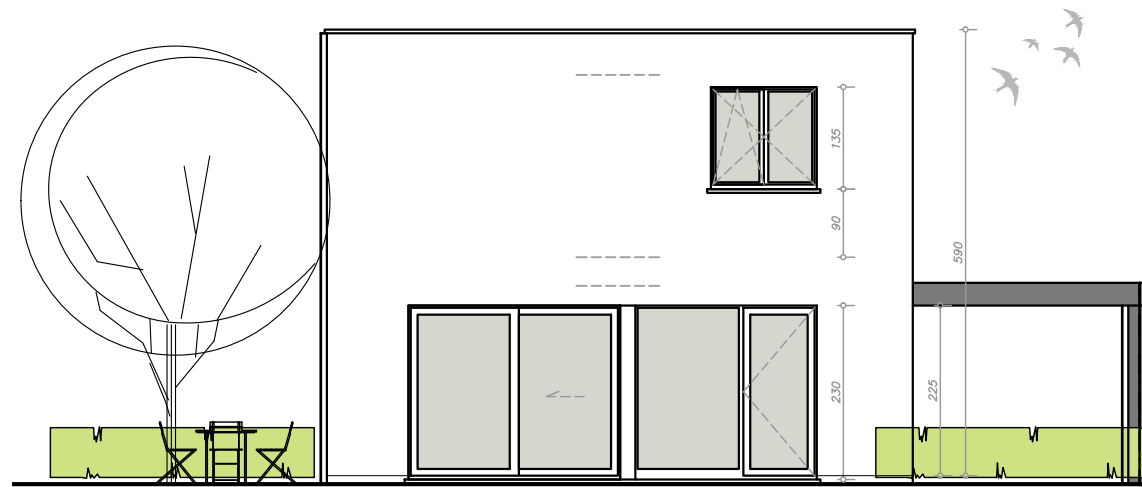
ACHTERGEVEL
