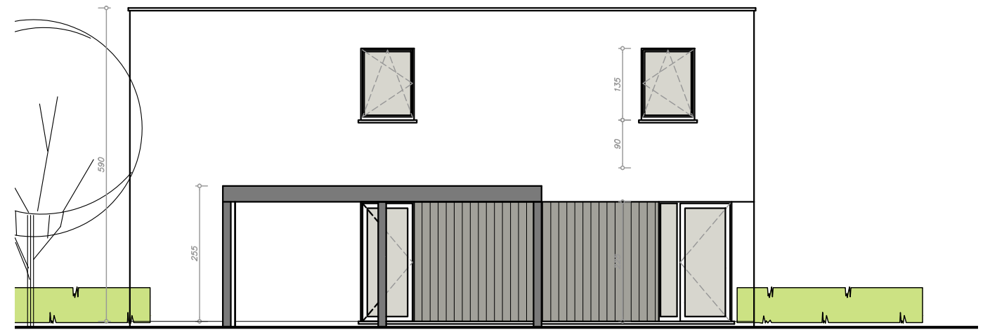
ZIJGEVEL LINKS
