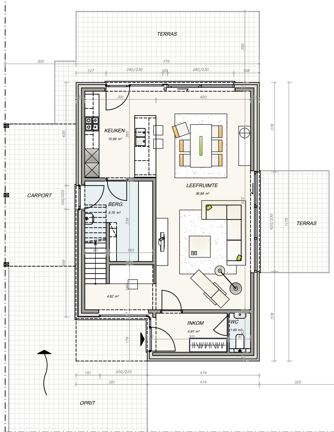
lot 37 (opp 86 m 2 excl. carport) GRONDPLAN
