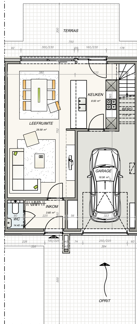
lot 24 (opp 75 m²) GRONDPLAN
