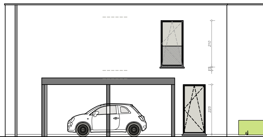
ZIJGEVEL LINKS
