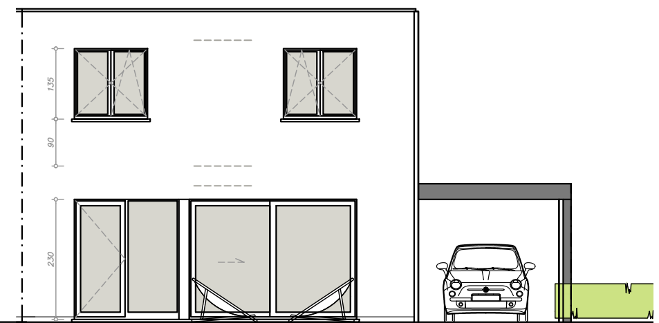
ACHTERGEVEL
