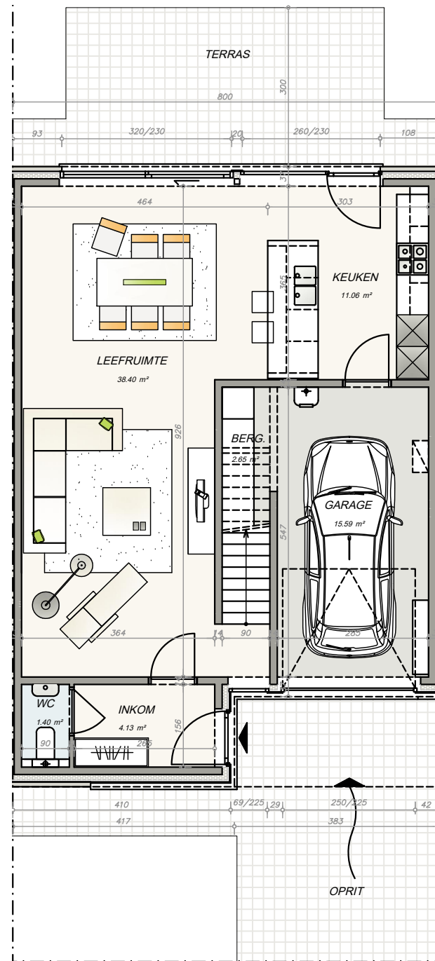
lot 20 (opp 87 m²) GRONDPLAN
