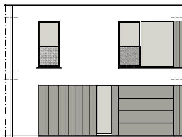
VOORGEVEL
