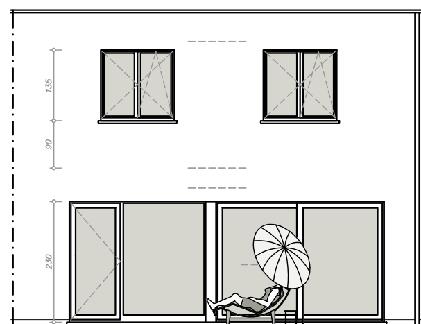
ACHTERGEVEL
